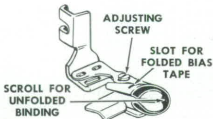
FIG. 69. THE BINDER.
