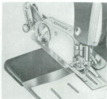
FIG. 84. THE BUTTONHOLER.
